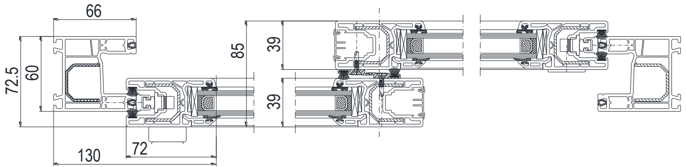
vízszintes metszet
