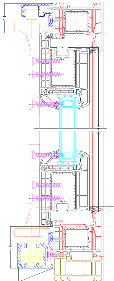
függőleges metszet
