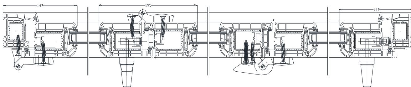
vízszintes metszet
